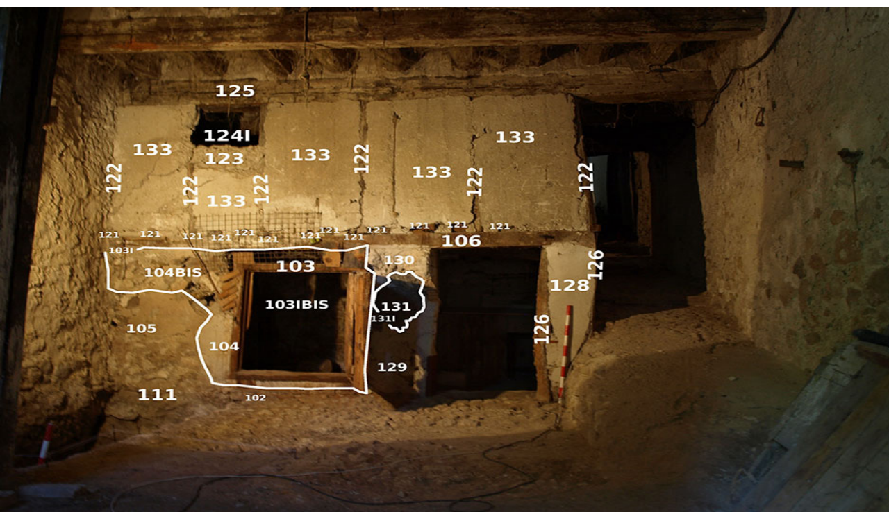
FIG. 14.- INDIVIDUALIZACIÓN SOBRE FOTOGRAFÍA DE LAS UNIDADES ESTRATIGRÁFICAS MURARIAS DE UNA DE LAS PARTES DEL SÓTANO DE LA CALLE CABALLEROS 11. (FOTO: SANTIAGO D. DOMÍNGUEZ-SOLERA.)
