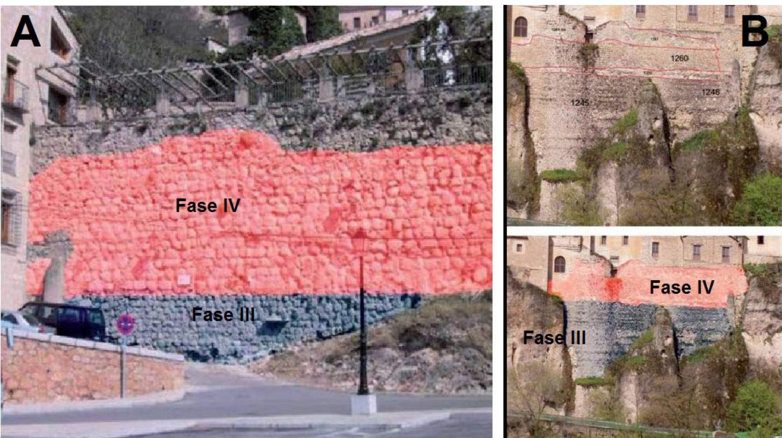
FIG. 5.- A = FASES III (ALFONSO VIII) Y IV (ALFONSO X) EN LOS LIENZOS DE MURALLA JUNTO AL ACTUAL COLEGIO DE ARQUITECTOS. B = LAS MISMAS FASES BAJO LA TRASERA DE LA CATEDRAL. (FOTOS: MÍCHEL MUÑOZ.)
