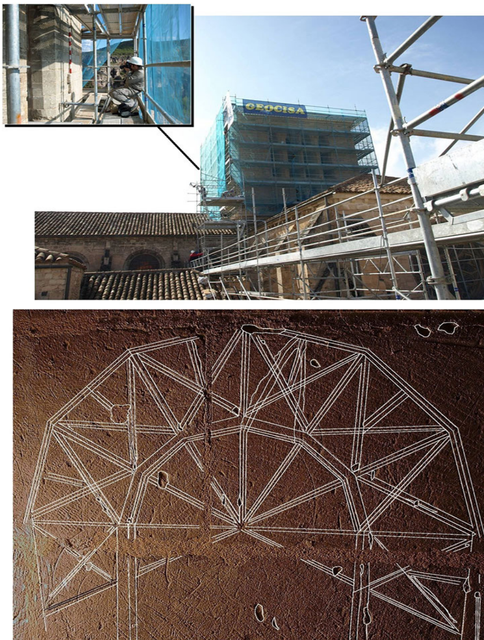
FIG. 23.- ARRIBA: TRABAJOS EN EL CIMBORRIO DE LA CATEDRAL DE CUENCA. (FOTOS: SANTIAGO D. DOMÍNGUEZ-SOLERA.) ABAJO: DIBUJO DE LA GIOLA DE UN TEMPLO ENCONTRADO EN EL CIMBORRIO DE LA CATEDRAL DE CUENCA. (LÁMINA: MÍCHEL MUÑOZ.)
